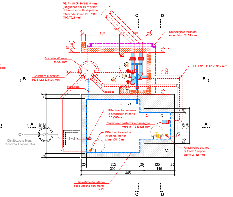
Pianta 3
