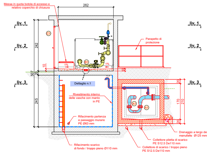
Sezione C-C
