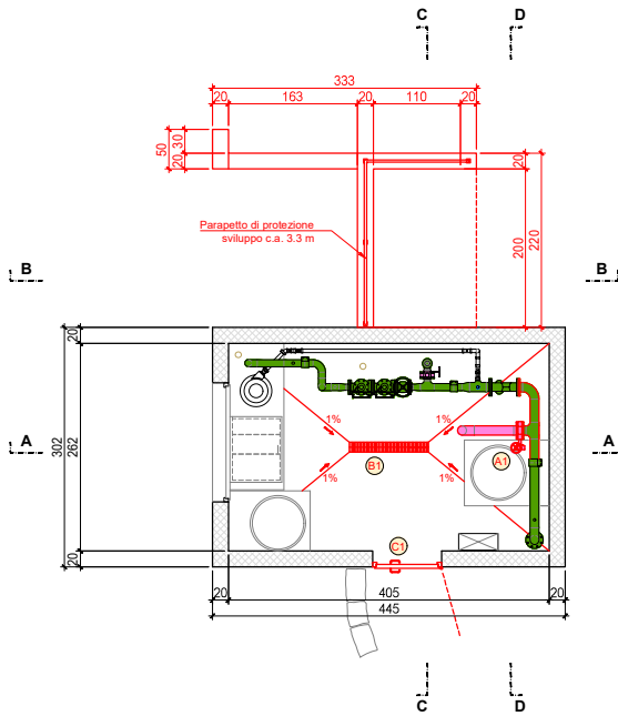
Pianta 1
